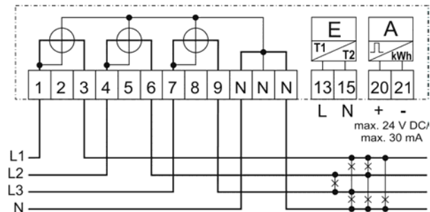
Licznik dwutaryfowy z wyjściem impulsowym SO
