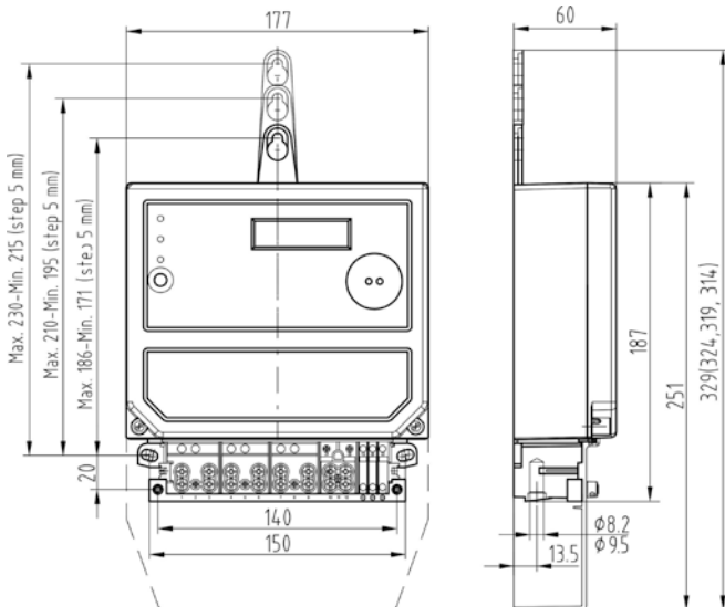
Пуздро „E“ до 100 А с отверстием в клеммах \varnothing 8,2 мм Пуздро „9“ до 120 А с отверстием в клеммах \varnothing 9,5 мм
