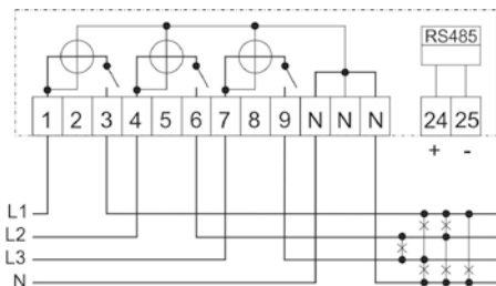
Прямое подключение с переключателем и интерфейсом RS 485
