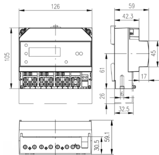
Корпус „C“ до 65 А с отверстием в клеммах \varnothing 6 мм
