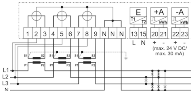
Полукосвенное подключение с внешним управлением тарифов, с импульсными выходами энергии +А и -А
